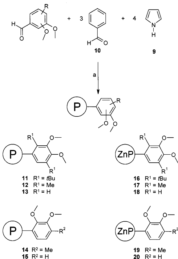
Scheme 2. a: BF 3 Et 2 O/CH 2 Cl 2 , room temp., DDQ
