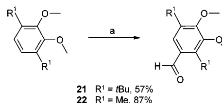
Scheme 3. a: Cl 2 CH-OMe, TiCl 4 , CH 2 Cl 2 , 0 °C
